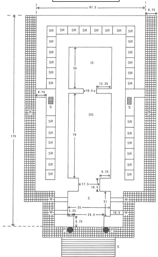
聖所的平面圖
