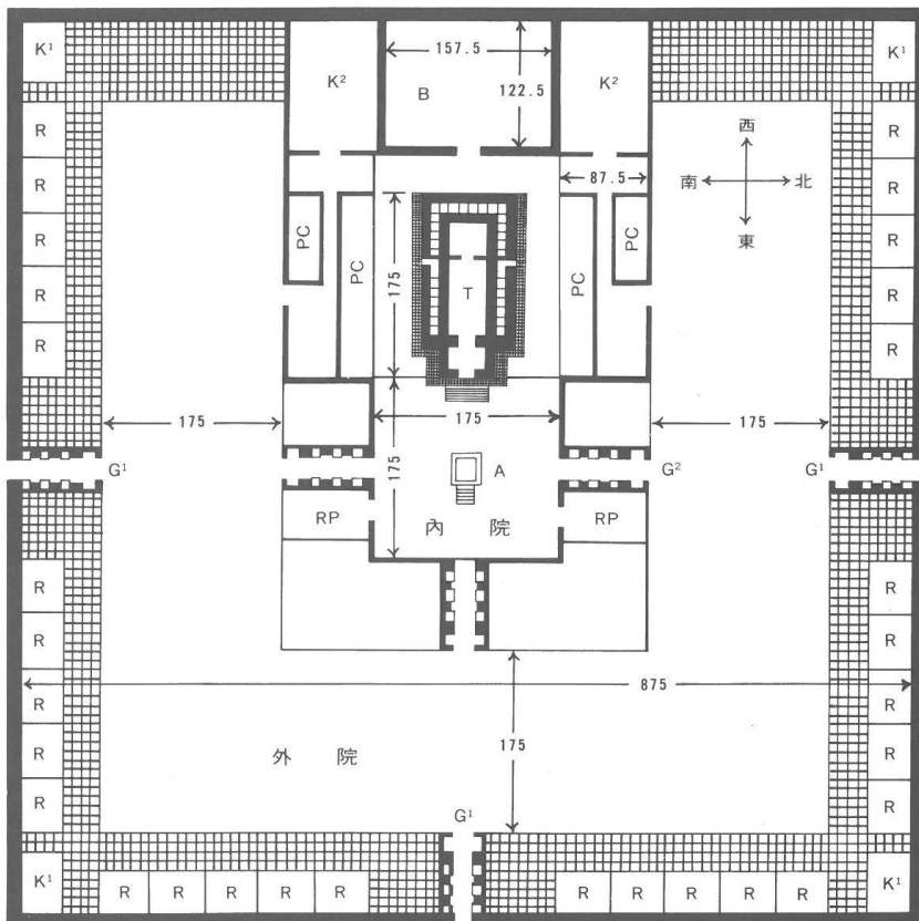
聖殿的平面圖
